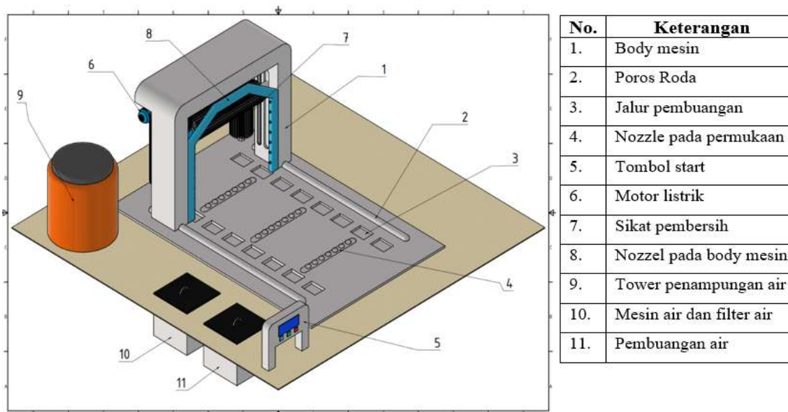
Gambar 4. Layout rancangan mesin pencuci mobil otomatis
