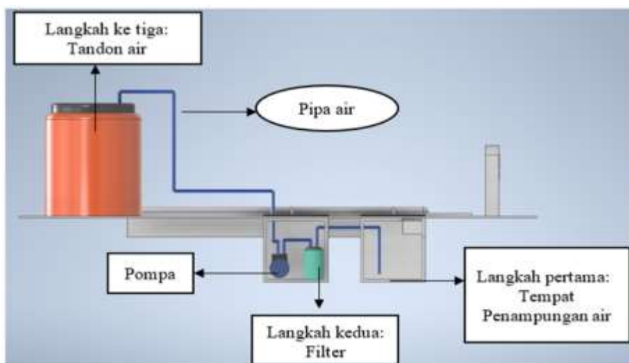
Gambar 5. Layout rancangan sistem sirkulasi air
