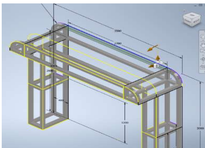
Gambar 2. Frame generator rancangan
