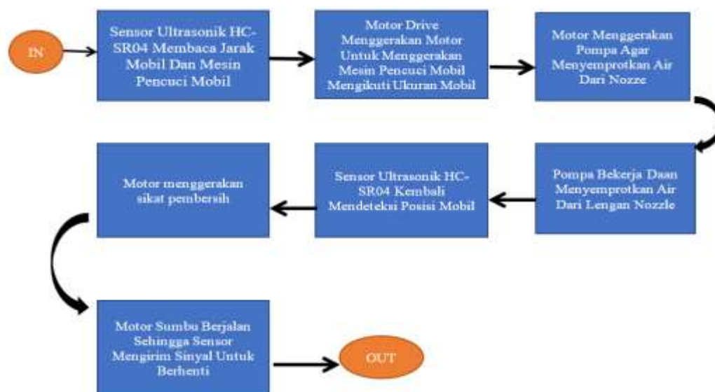
Gambar 6. Sistem operasi control dengan Arduino
