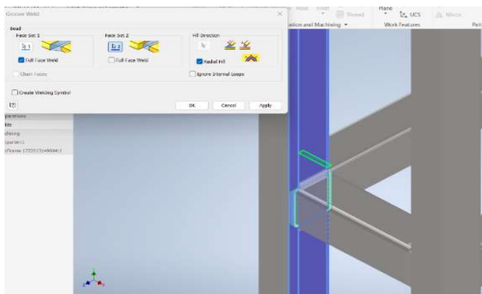
Gambar 3. Rancangan pengelasan rangka
